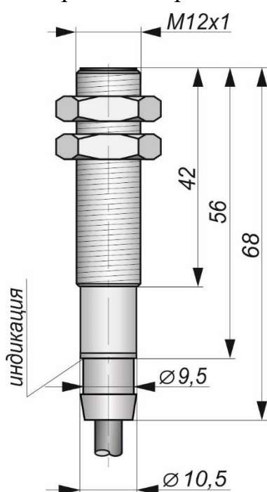
Габаритный чертеж
